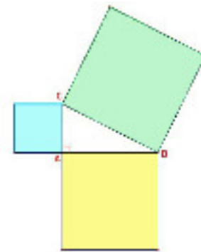
Pythagore BC^2 = BA^2 + AC^2 600 av J.C.
